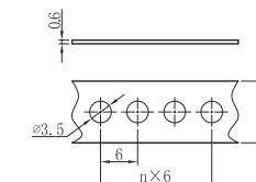
UJ5-2.5WNE монтаж
